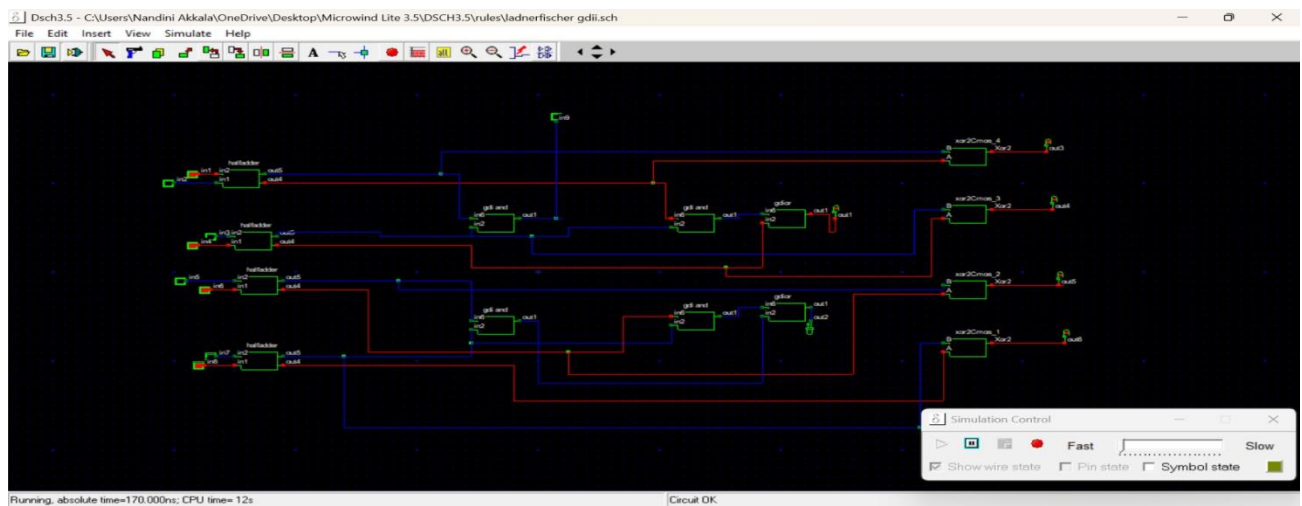
Fig 4 : GDI Ladner Fischer Prefix Adder
