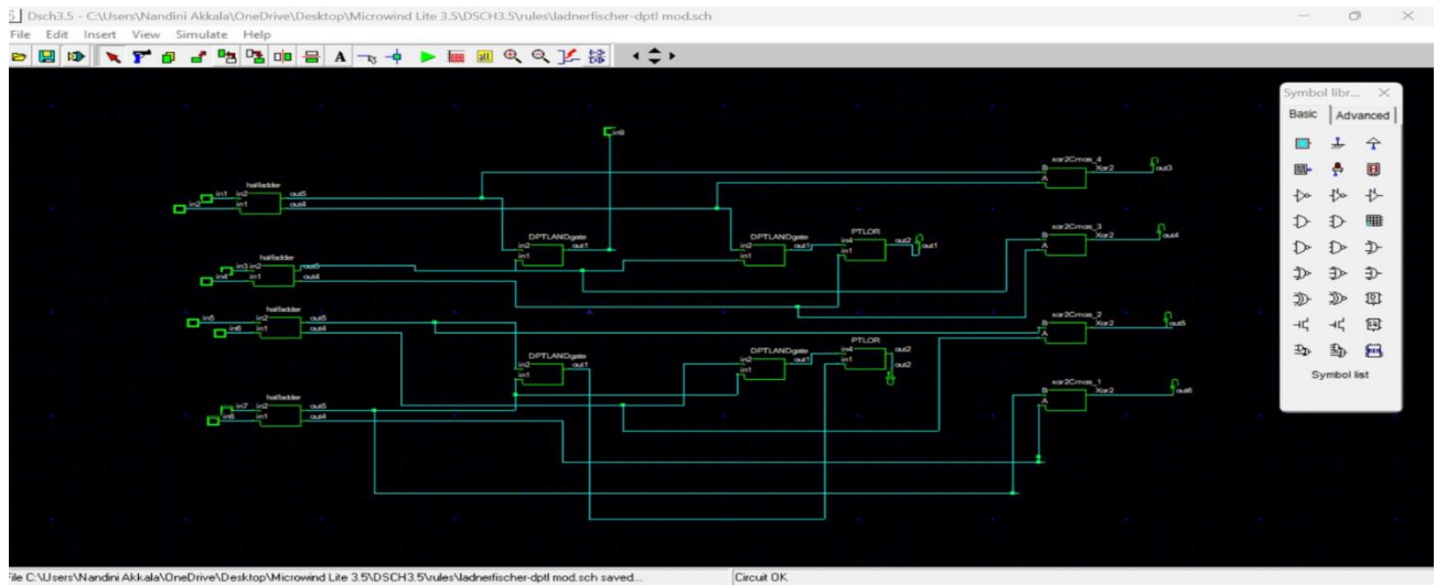
Fig 3 : DPTL Ladner Fischer Prefix Adder
