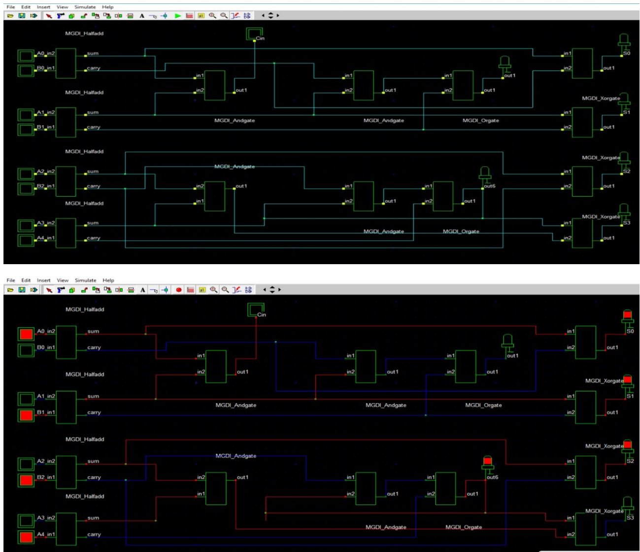
Fig 5 : MGDI Ladner Fischer Prefix Adder
