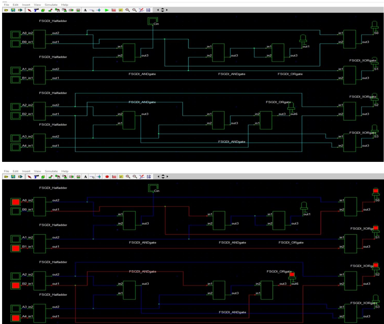
Fig 6 : FSGDI Ladner Fischer Prefix Adder
